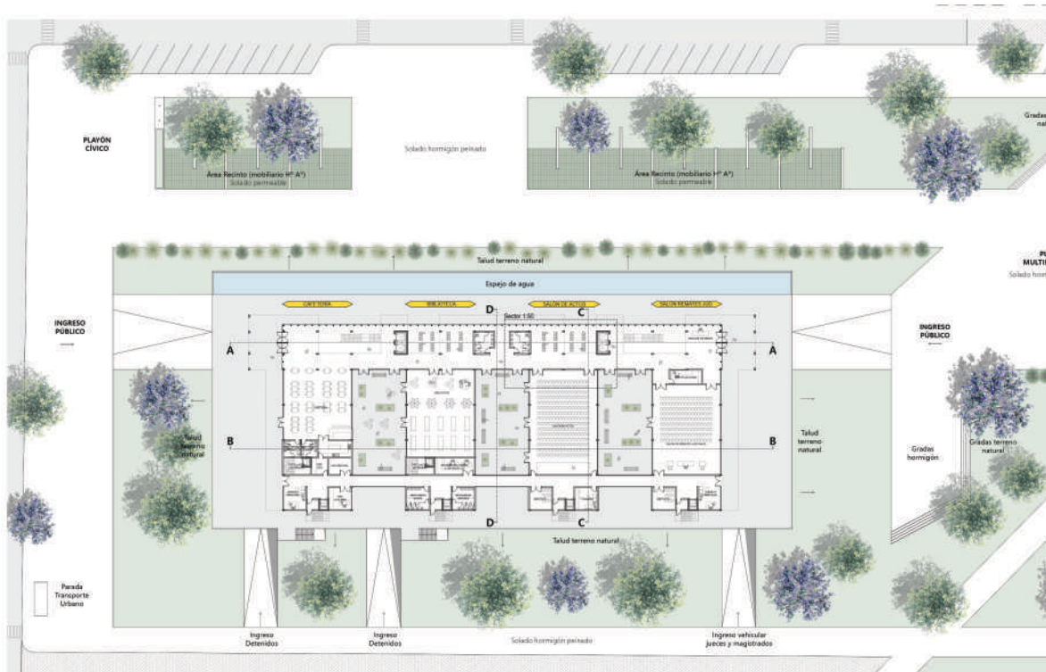
Planta Baja Esc. 1:200
